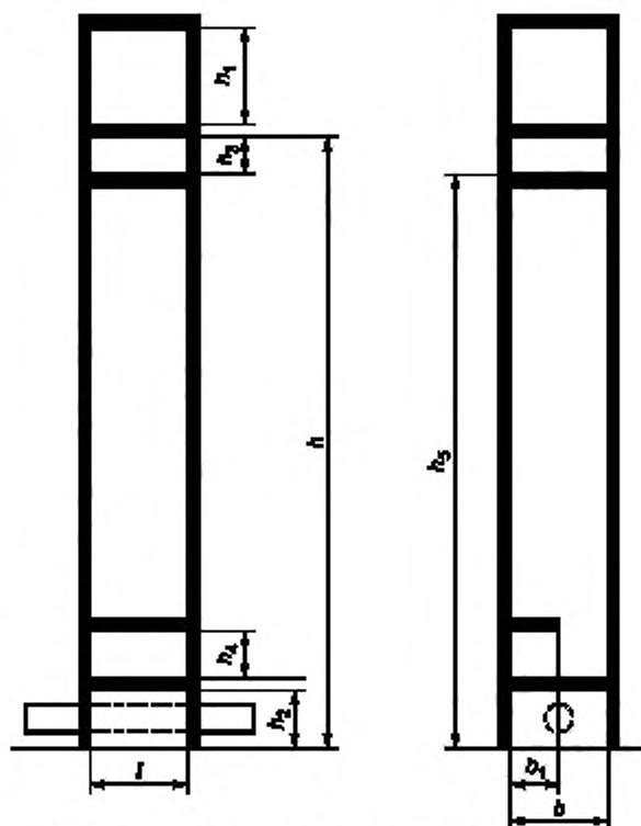
Рисунок 8 — Шкаф для детской одежды (от 3 до 7 лет)
