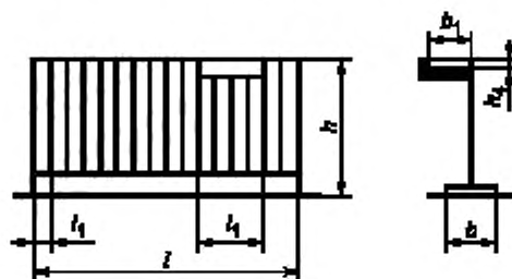
Рисунок 16 — Барьер
