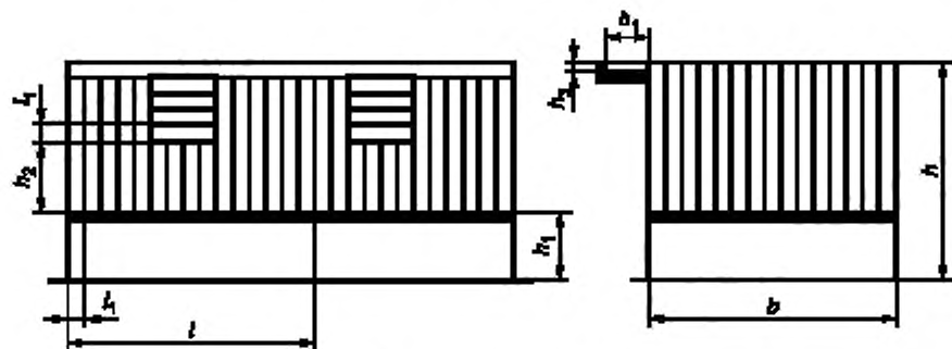
Рисунок 15 — Манеж общий (с 5 до 9 мес)
