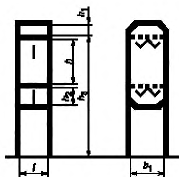
Рисунок 18 — Напольная вешалка
