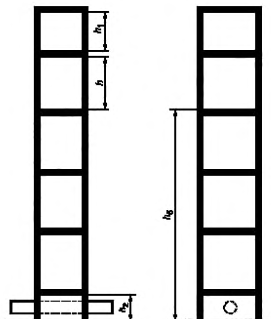
Рисунок 6 — Шкаф для детской одежды (до 9 мес. включ.)
