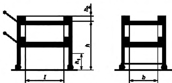
Рисунок 4 — Сервировочный стол
