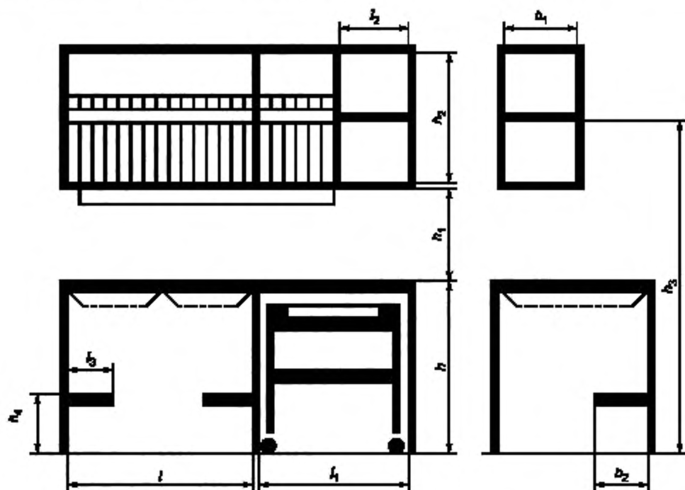
Рисунок 12 — Шкаф под мойку и для хранения посуды
