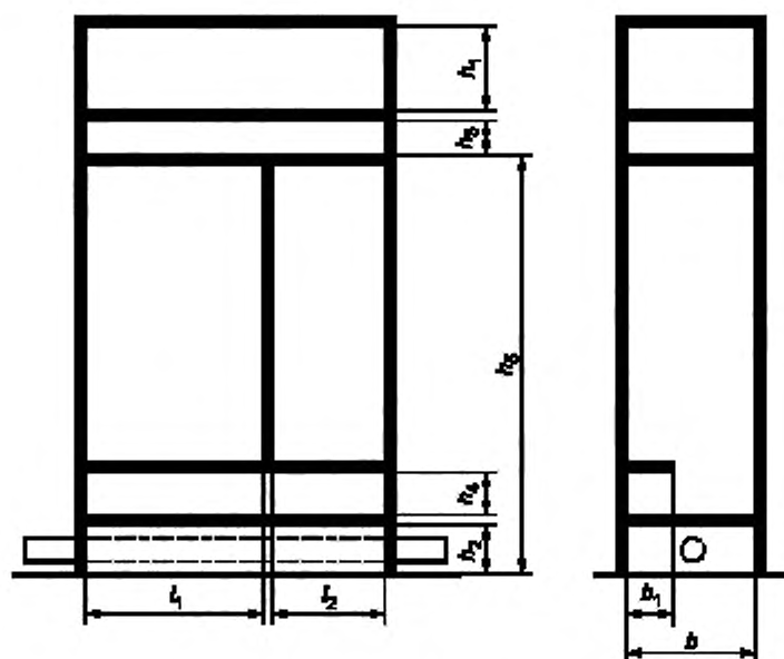
Рисунок 9 — Шкаф для одежды персонала
