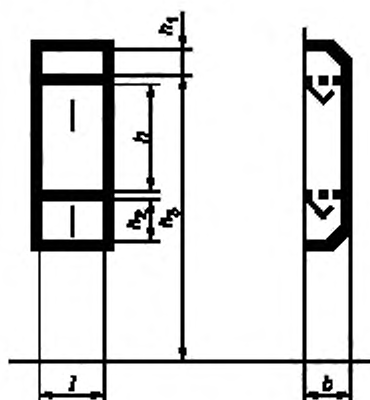
Рисунок 17 — Настенная вешалка
